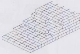
الشكل ١٤: تقنية رصف لبينات الرامشن (عن: Sauvage, M. 2016, fig. 7).
