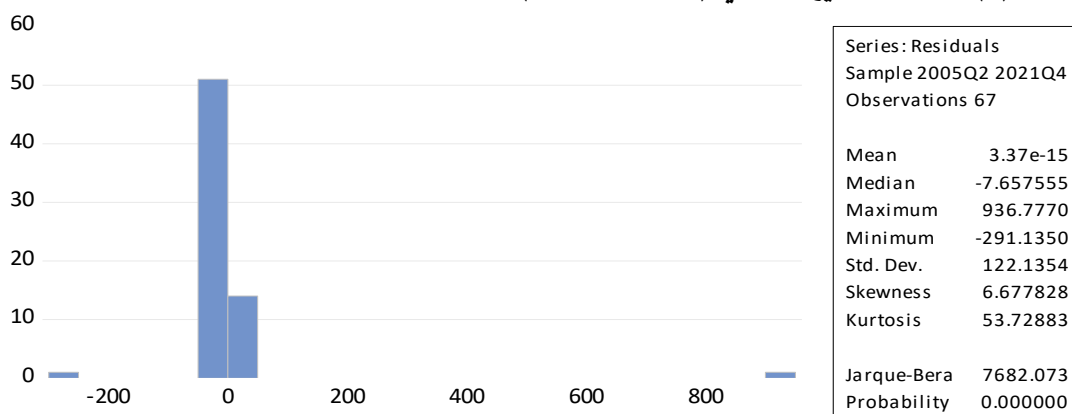
الشكل (٣): اختبار التوزيع الطبيعي (Jarque-Bera)
