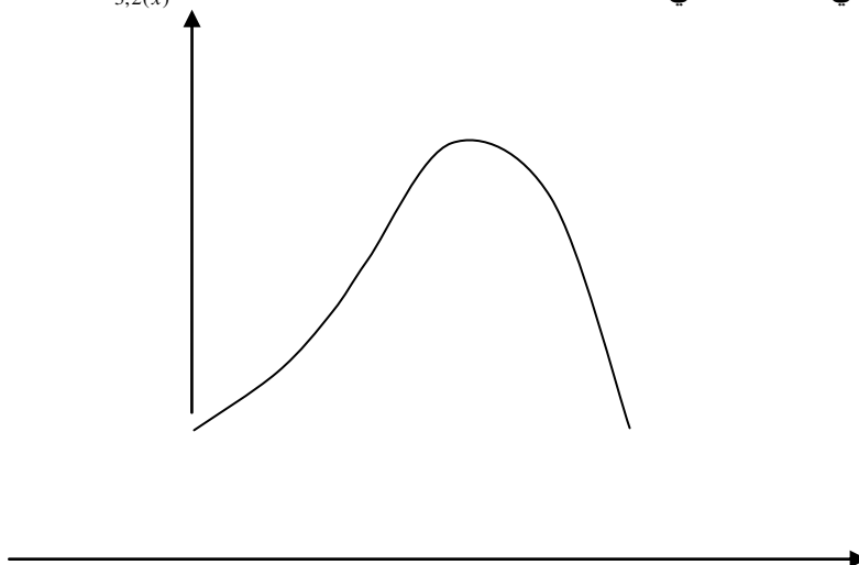
الشكل البياني رقم (3) للتوزيع المعياري B_{3,2}(x)
