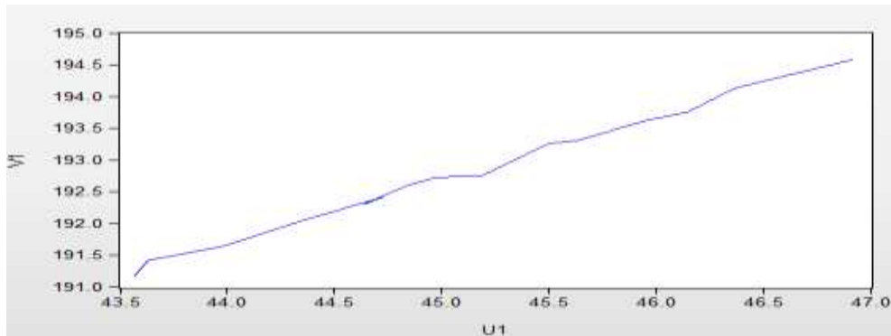
الشكل رقم (3) الشكل البياني بين المركبين القانونيين الخام U1 و V1
