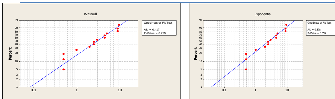
الشكل (4) الرسم الاحتمالي ونتائج اختبار (A-D) لأزمنة الإصلاح لآلة الغزل المصدر: إعداد الباحثة استناداً لبيانات فترات الإصلاح الواردة في الجدول (6) باستخدام برنامج MINITAB
