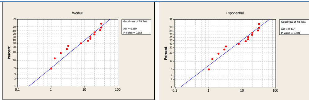
الشكل (3) الرسم الاحتمالي ونتائج اختبار (A-D) لأزمنة العمل لآلة الغزل المصدر: إعداد الباحثة استناداً لبيانات فترات العمل الواردة في الجدول (6) باستخدام برنامج MINITAB
