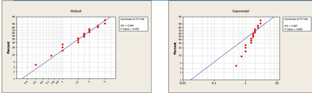
الشكل (10) الرسم الاحتمالي ونتائج اختبار (A-D) لأزمنة الإصلاح لآلة التدوير
