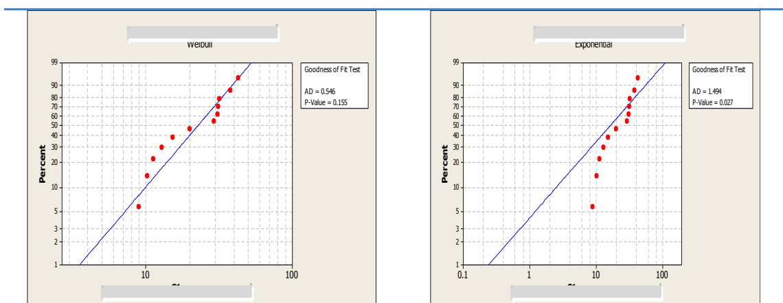
الشكل (1) الرسم الاحتمالي ونتائج اختبار (A-D) لفترات العمل لآلة الكرد
