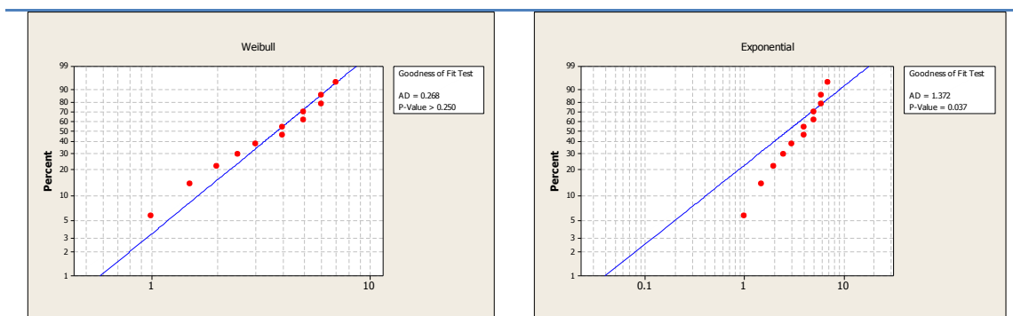
الشكل (2) الرسم الاحتمالي ونتائج اختبار (A-D) لفترات الإصلاح لآلة الكرد
