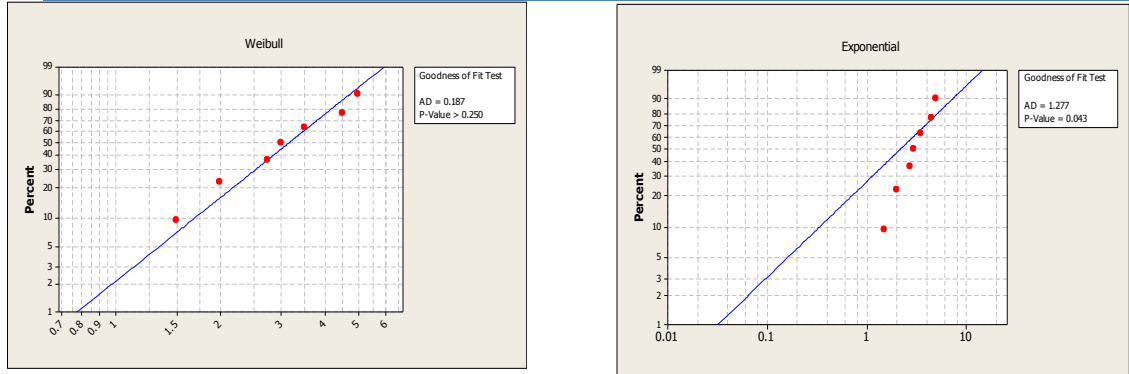
الشكل (8) الرسم الاحتمالي ونتائج اختبار (A-D) لأزمنة الإصلاح لآلة البرم
