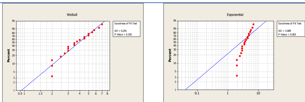
الشكل (6) الرسم الاحتمالي ونتائج اختبار (A-D) لأزمة الإصلاح لآلة السحب
