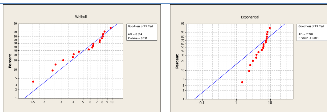
الشكل (9) الرسم الاحتمالي ونتائج اختبار (A-D) لأزمدة العمل لآلة التدوير
