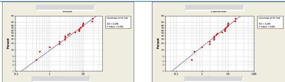
الشكل (5) الرسم الاحتمالي ونتائج اختبار (A-D) لأزمنة العمل لآلة السحب
