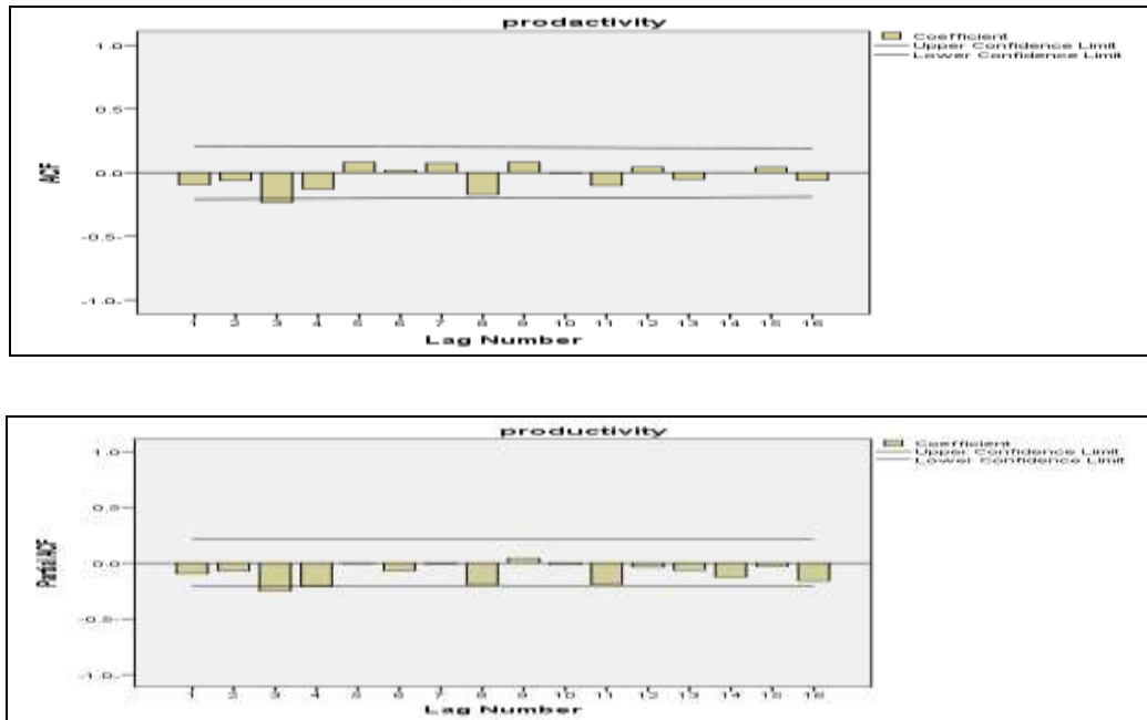
الشكل (4) دالتي الارتباط الذاتي والارتباط الذاتي الجزئي بعد أخذ الفروق لمرة واحدة
