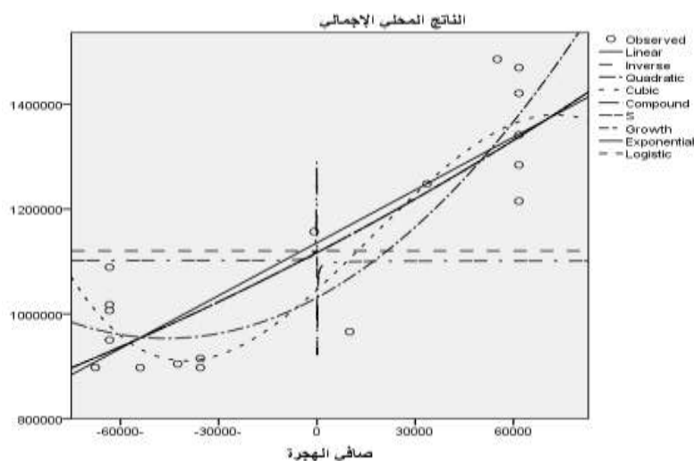
الشكل (1): منحنيات توابع تمثيل العلاقة بين الناتج المحلي الإجمالي وصافي الهجرة
