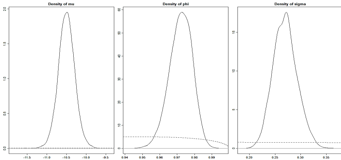
الشكل (6): التوزيعات الاحتمالية اللاحقة لمعاملات نموذج التقلب العشوائي (الخط متصل) والتوزيعات السابقة (الخط المنقطع).
