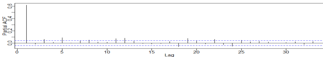
الشكل (3): دالة الارتباط الذاتي والجزئي لعوائد سوق دمشق للأوراق المالية.
