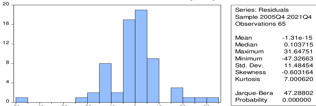
الشكل (٣): اختبار التوزيع الطبيعي للبواقى (Jarque-Bera)
