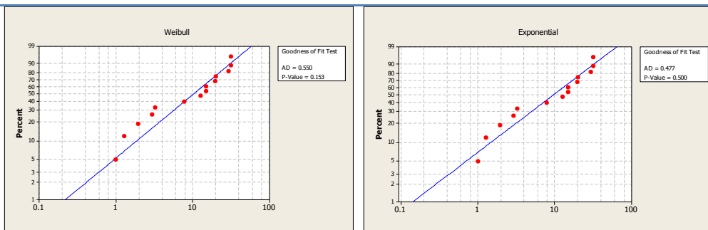
الشكل (3) الرسم الاحتمالي ونتائج اختبار (A-D) لأزمنة العمل لآلة الغزل المصدر: إعداد الباحثة استناداً لبيانات فترات العمل الواردة في الجدول (6) باستخدام برنامج MINITAB
