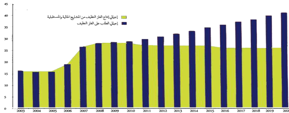
الشكل رقم: (5): توقعات إجمالي الطلب على الغاز النظيف من المشاريع المحلية المنفذة والمتوقعة تنفيذها (مليون م³ يومياً)
